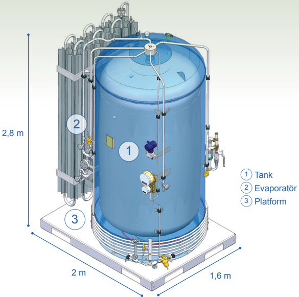
3.000 L Skid Tank
